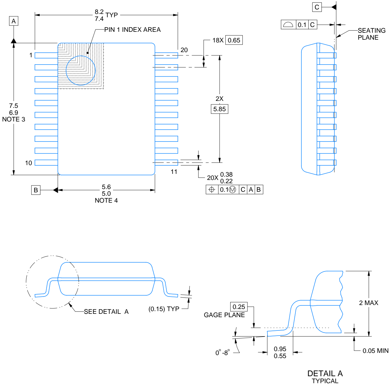
图 8 SSOP20 封装尺寸信息
