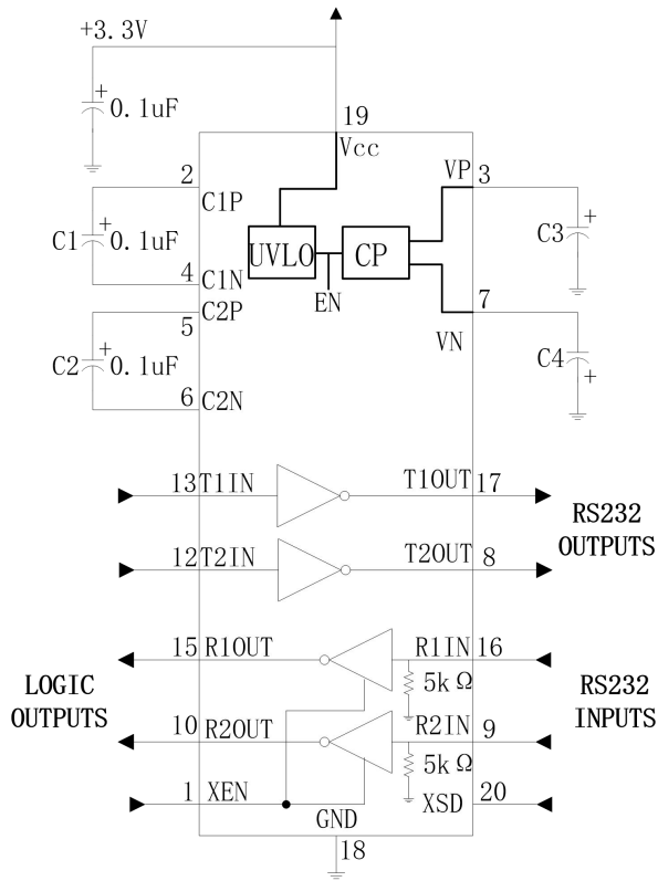
图 6 ASRS3222E 典型外围应用电路
