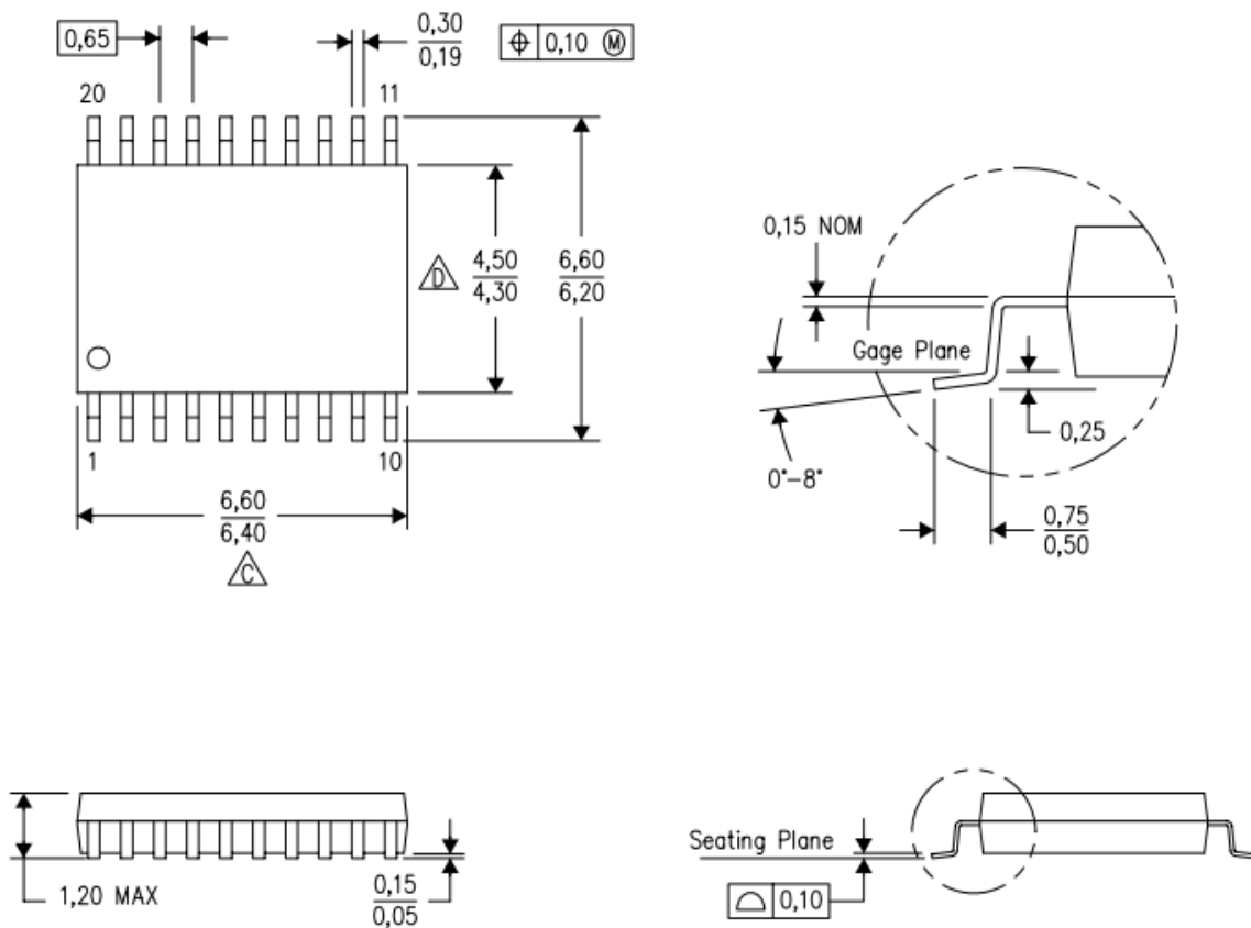
图 7 TSSOP20 封装尺寸信息
