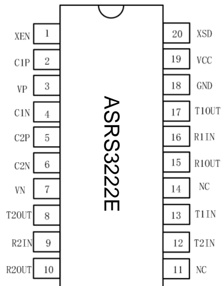
ASRS3222E 引脚图—20-pin SSOP20/TSSOP20
